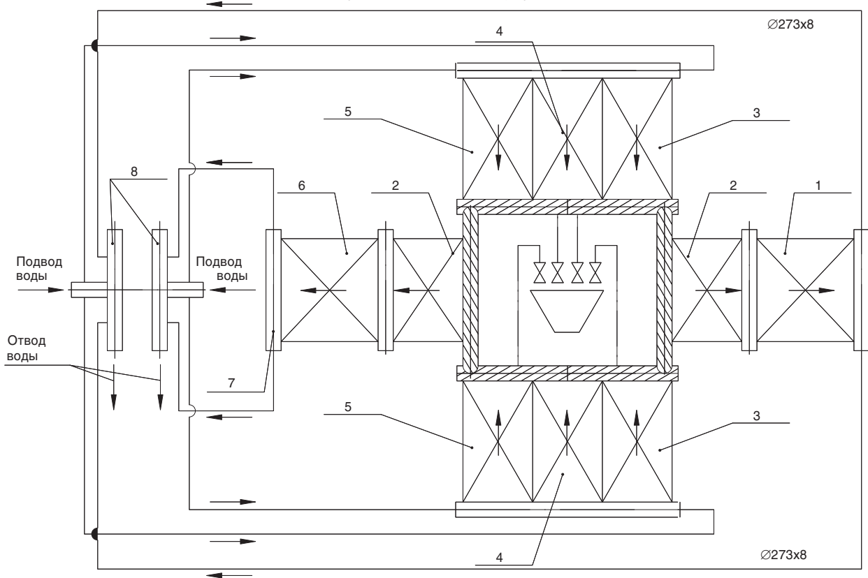
Двухходовая схема циркуляции
