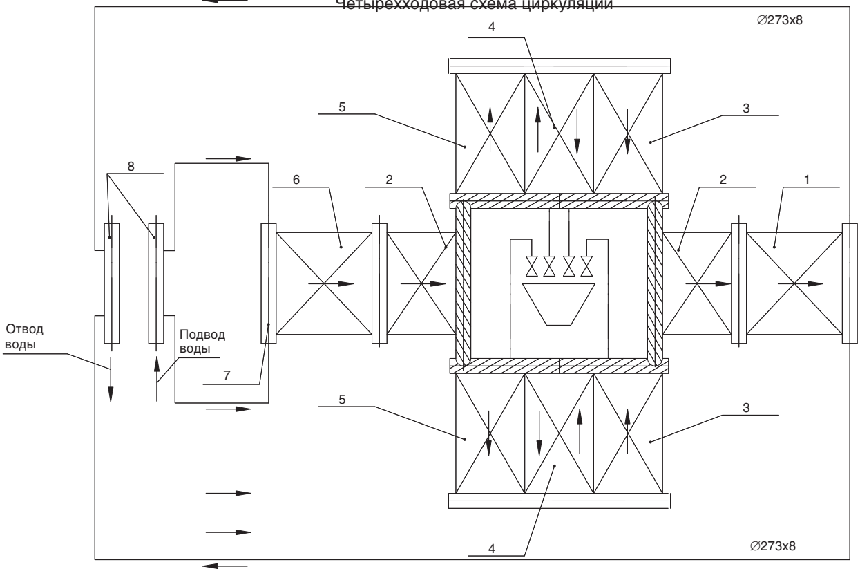
Четырехходовая схема циркуляции
