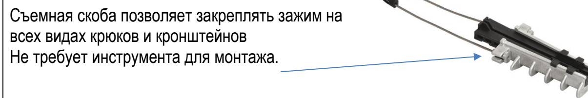
Зажим анкерный ЗАН 50-70/1500 клинового типа
