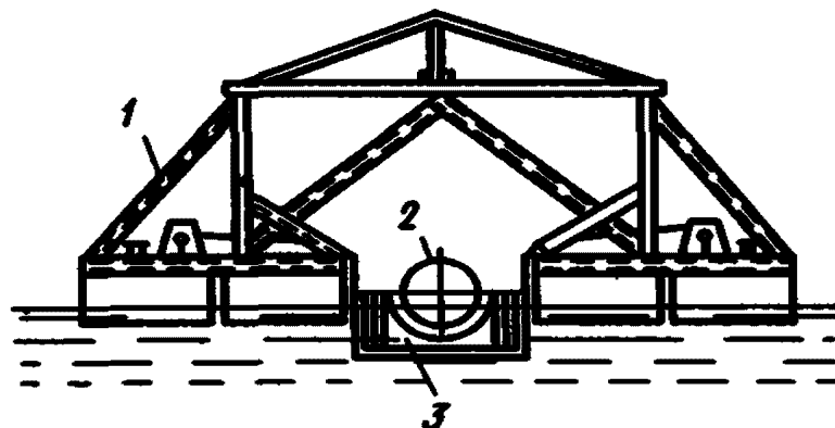
Рис. 1. Схема установки плавучей камеры для сварки межсекционного стыка: 1 — плавучая порталная опора; 2 — трубопровод; 3 — плавучая камера
