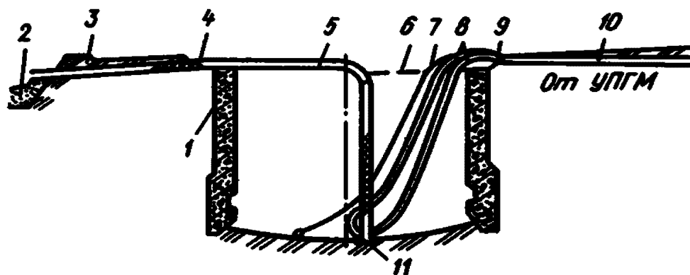
Рис. 2. Схема разработки грунта при опускании колодца насосной станции средствами гидромеханизации: 1 — стенка колодца насосной станции; 2 — отвал грунта, 3 — пульпопровод; 4 — гибкий отводящий шланг; 5 — система труб и отводящих шлангов для подъема пульпы; 6 — система тросов, удерживающих отводящие шланги и трубы; 7 — напорный шланг к насадке; 8 — система гибких напорных шлангов к гидроэжектору; 9 — распределительное устройство; 10 — напорный трубопровод от УПГМ-360; 11 — гидроэжектор
