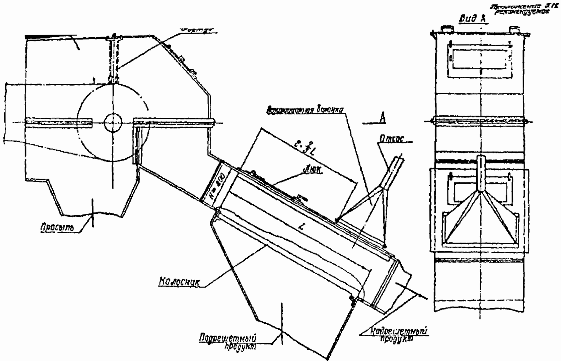
Укрытие неторбожного колосникового грохота
