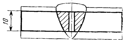
Дуговая сварка
