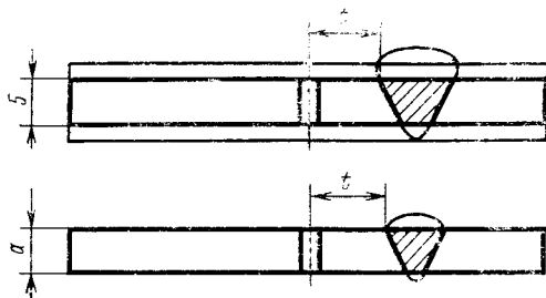
Дуговая сварка
