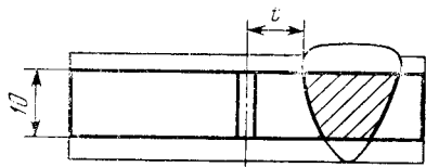
Дуговая сварка
