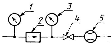
Схема определения расходных характеристик предохранительных устройств
