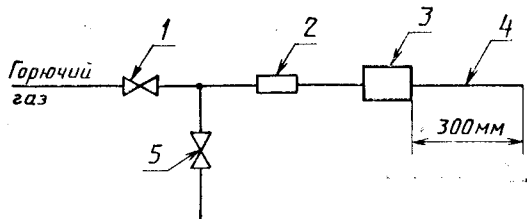
Схема испытания отсечных клапанов, срабатывающих от температуры
