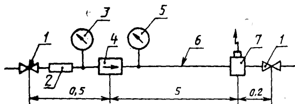
Схема испытаний пламепреграждающих устройств Размеры в метрах
