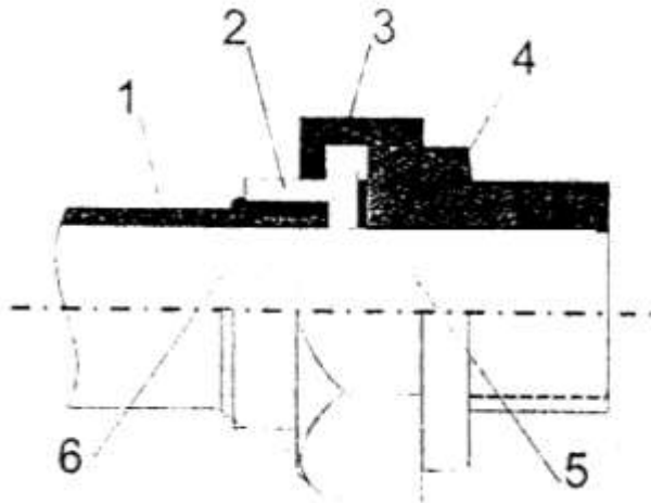
Рис. 5.4. Соединение с накладной гайкой
