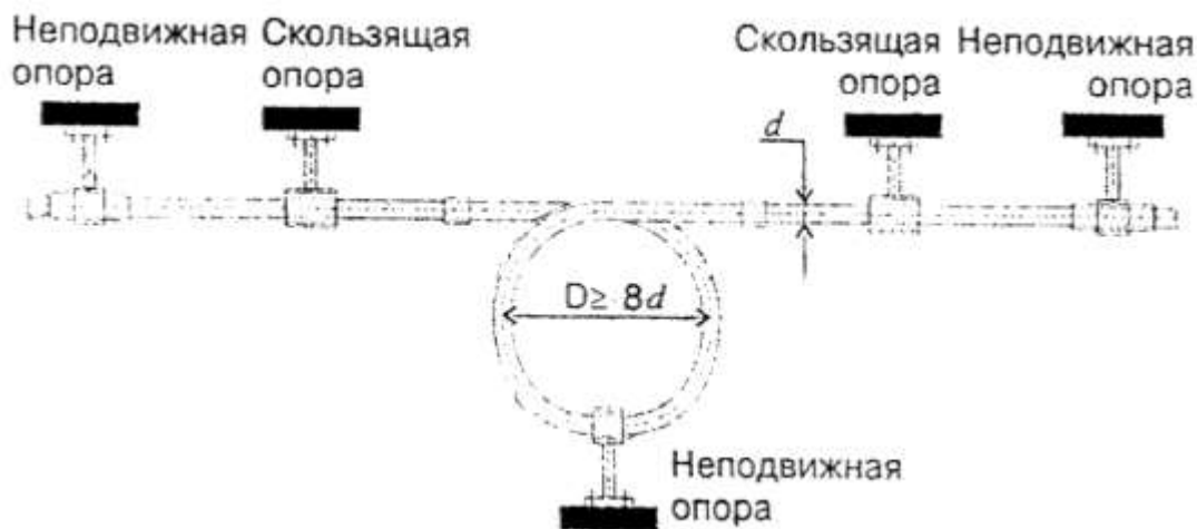
Рис. 2.6. Петлеобразный компенсатор
