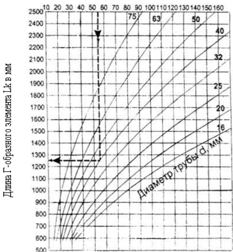
Рис. 2.7. Номограмма для определения длины участка трубы, воспринимающего тепловое удлинение
