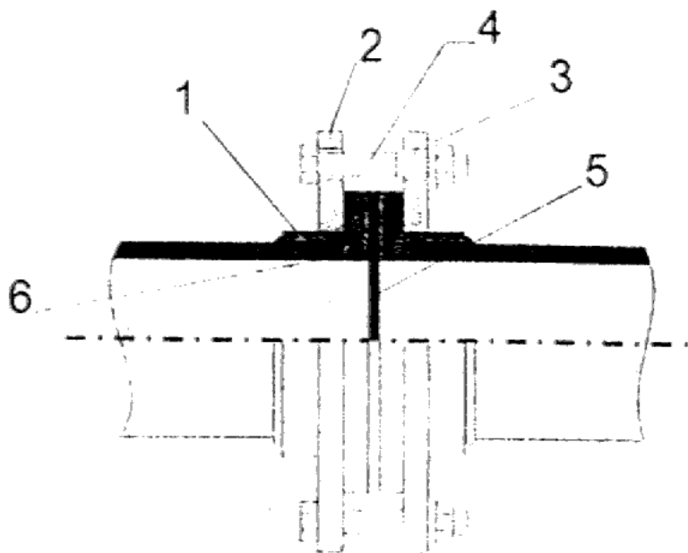
Рис. 5.3. Соединение труб из PPRC на свободных фланцах
