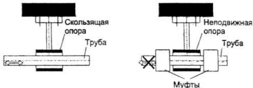
Рис. 4.1. Виды опор
