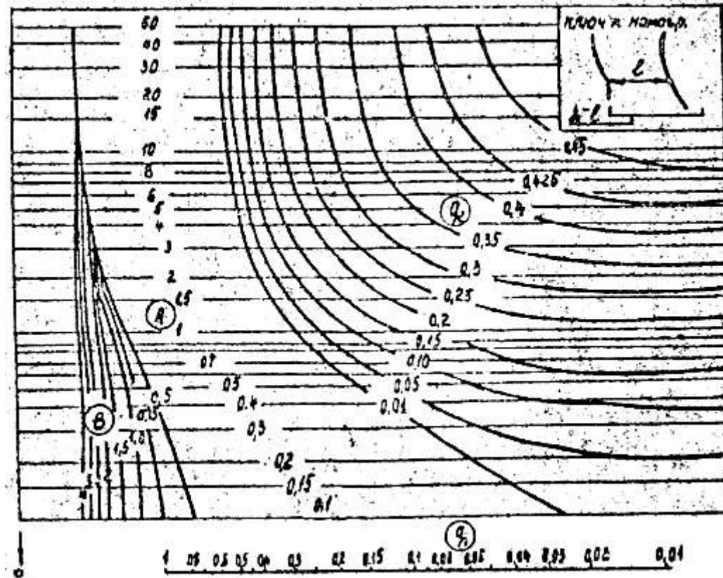
Рис. 3.2. Номограмма для определения R
