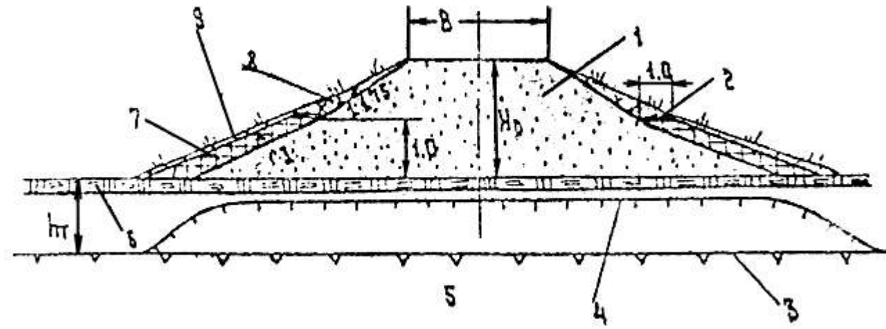
Конструкции земляного полотна промышленных железных дорог
