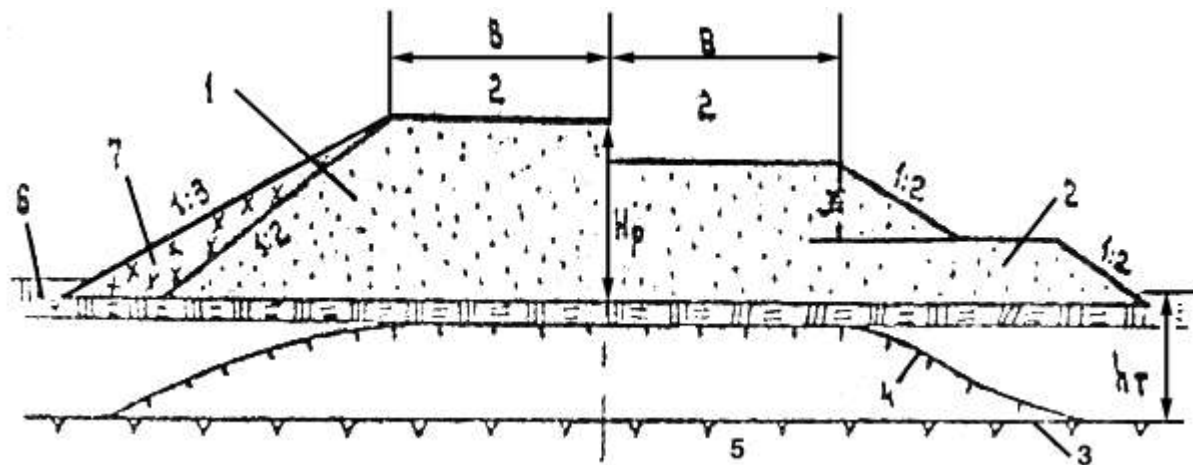
Конструкции земляного полотна подъездных автомобильных дорог промышленных предприятий
