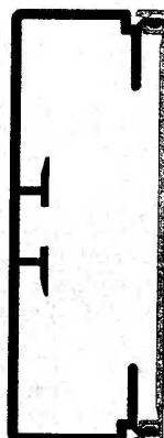
CM110x40 №17614
